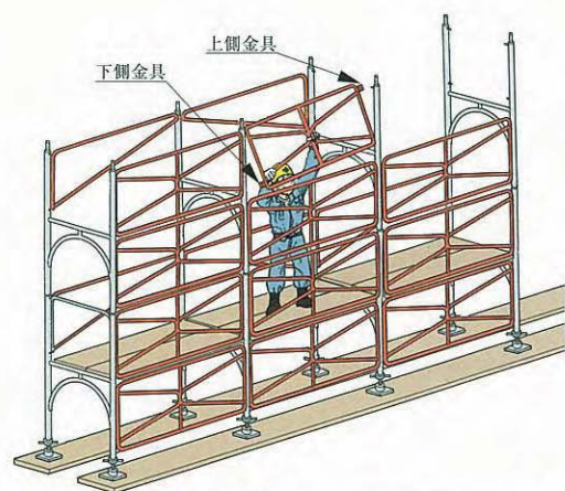
手すり先行専用足場方式の例
